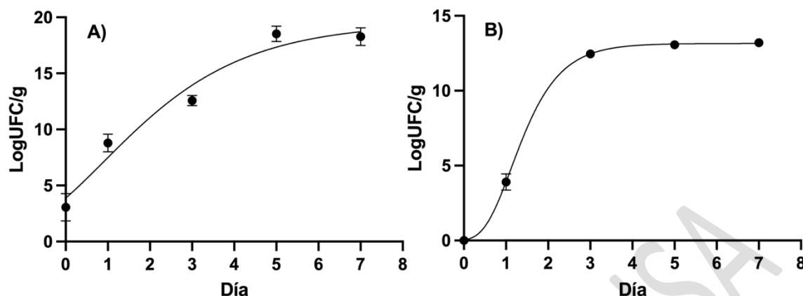
Fig. 1. Cinética de crecimiento microbiológico de la masa madre. Los valores representan la media \pm SD (n=3) (A) LAB. (B) Levaduras.
