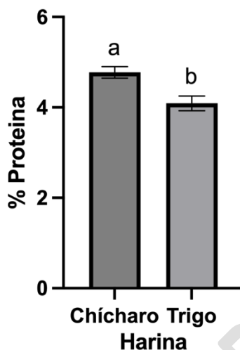
Fig. 3. Comparación del % de proteína entre la harina de chícharo y la de trigo. Los valores representan la media \pm SD (n=3).
