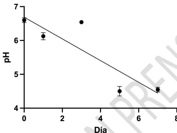
Fig. 2. Disminución del pH durante la fermentación. Los valores representan la media \pm SD (n=3)
