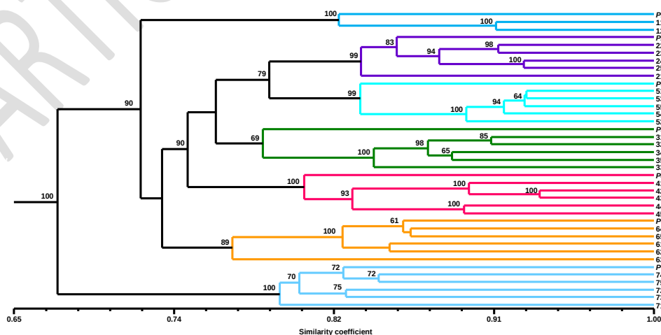
Figura 1. Dendrograma que muestra las relaciones genéticas entre plantas madre y sus
