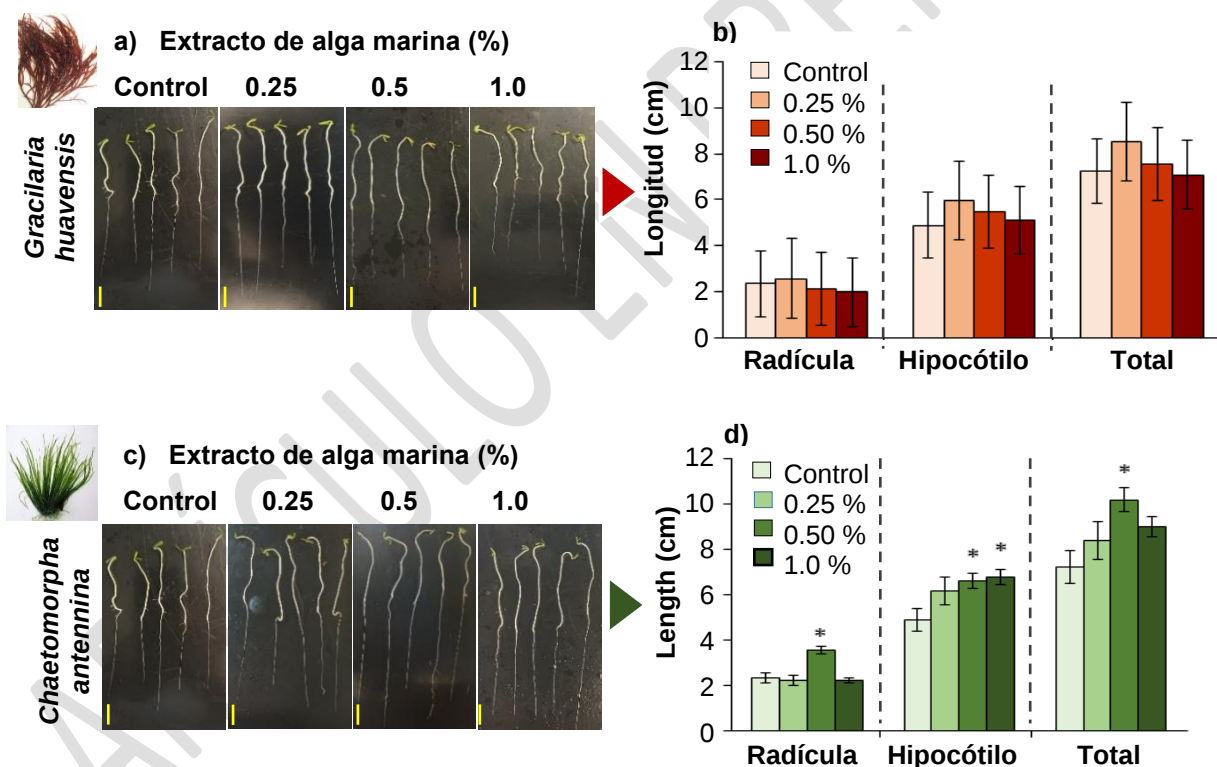
Figura 1. Efecto de los extractos de (a,b) Gracilaria huavensis y (c,d) Chaetomorpha antennina a concentraciones de 0.25, 0.5 y 1.0 % en la longitud de la radícula, hipocótilo y total. (Barra = 1 cm)
