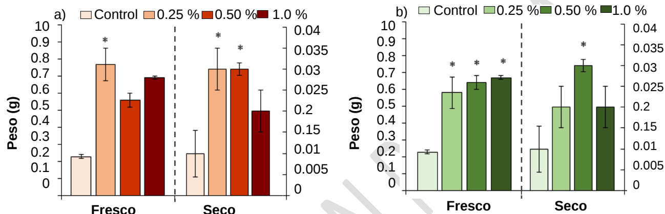
Figura 2. Efecto de los extractos acuosos de (a) Gracilaria huavensis y (b) Chaetomorpha antennina a concentraciones de 0.25, 0.5 y 1.0 % en el peso fresco y seco de las plántulas de jitomate
