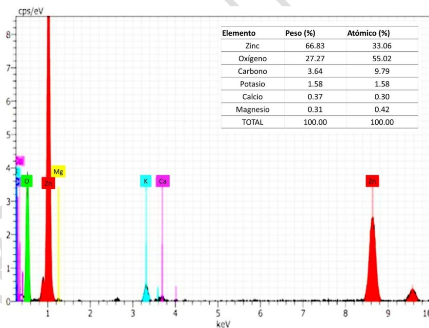
Figura 2. Espectro EDX de la síntesis de NPs ZnO usando extracto de flor de Tithonia diversifolia
