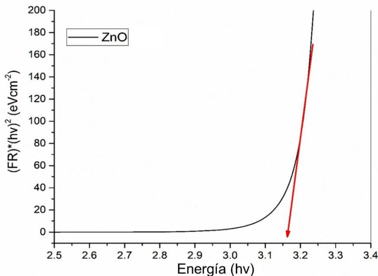
Figura 3. Cálculos de Bandgap para nanopartículas de ZnO
