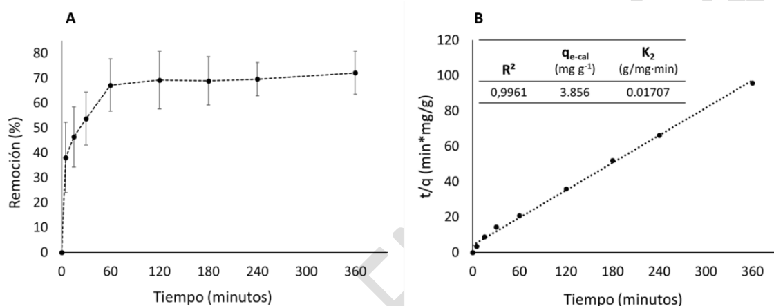
Figura 1. Adsorción de As por BG en función del tiempo. A) Porcentaje de remoción en el tiempo. B) Ajuste lineal del modelo pseudo-segundo orden, de la adsorción en diferentes tiempos. Se muestran los parámetros cinéticos calculados. R^2 : coeficiente de correlación; q_{e-cal} : cantidad máxima de As que el biocarbón puede adsorber cuando se alcanza el equilibrio; K_2 : constante de velocidad de pseudo-segundo orden. Fuente: Elaboración propia a partir de los resultados.
