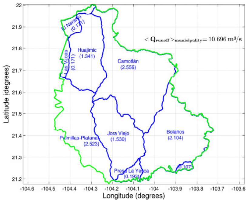
Figure 8. Average runoff volume ( \text{m}^3 \text{ s}^{-1} ), in La Yesca municipality. Figura 8. Volumen de escurrimiento medio ( \text{m}^3 \text{ s}^{-1} ) en el municipio de La Yesca.
