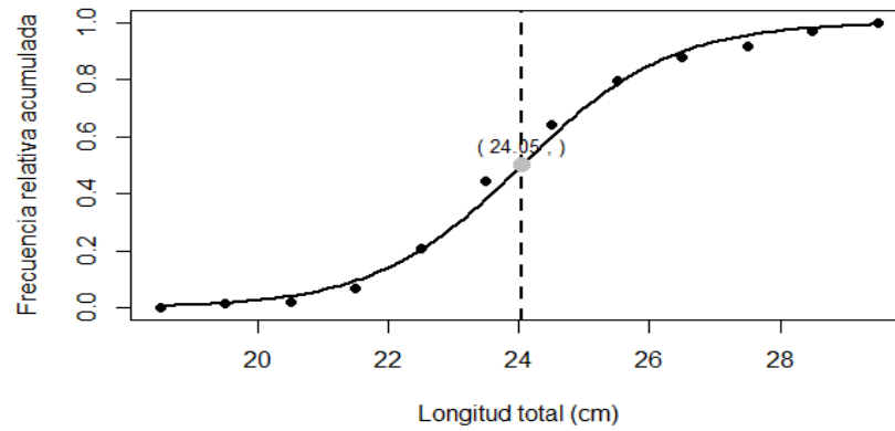
Figura 2. Talla media de captura de Mayaheros urophthalmus .
