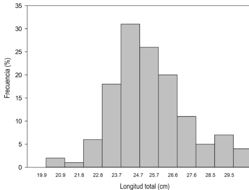
Figura 1. Estructura de tallas de Mayaheros urophthalmus .
